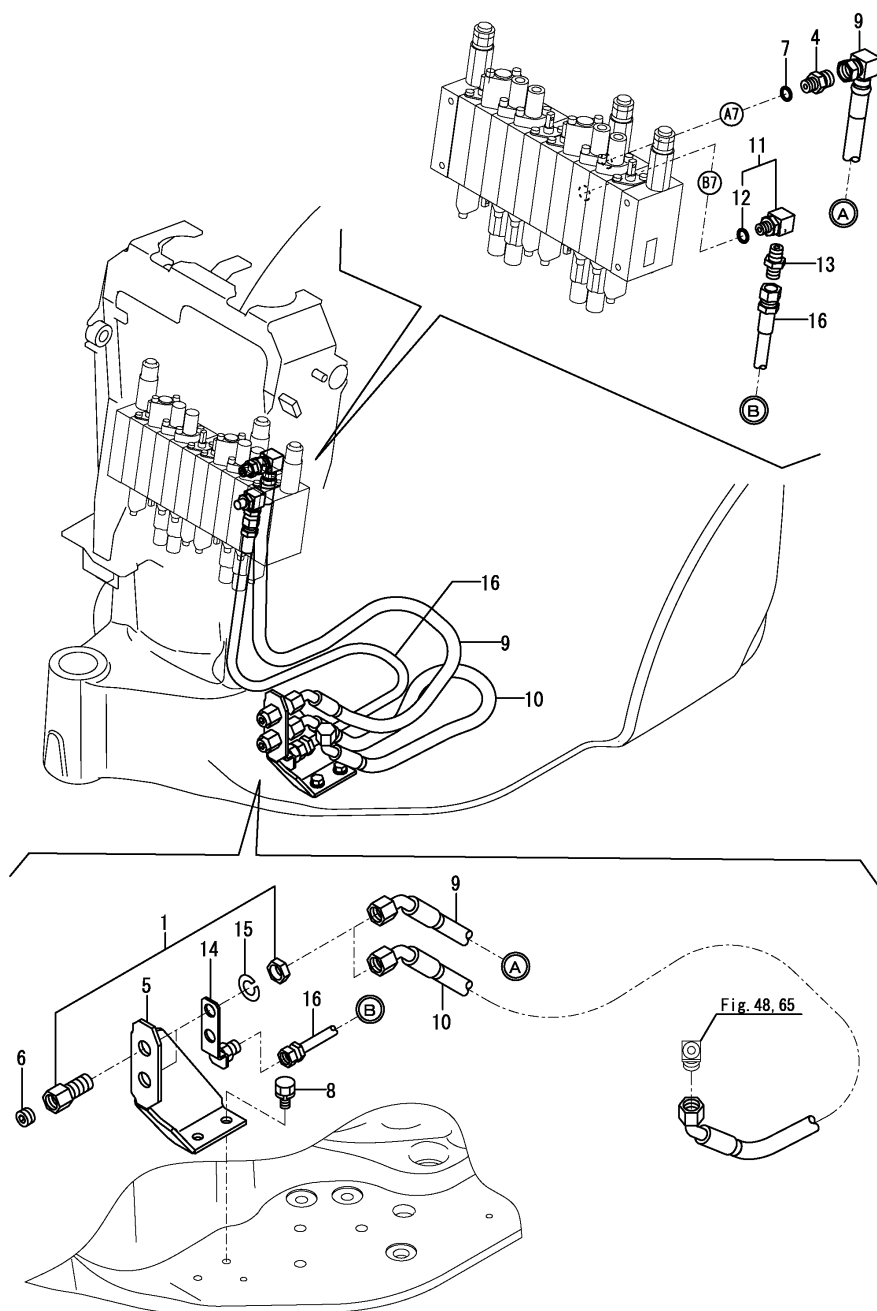
Fig.49. P.T.O.(FRAME END)
