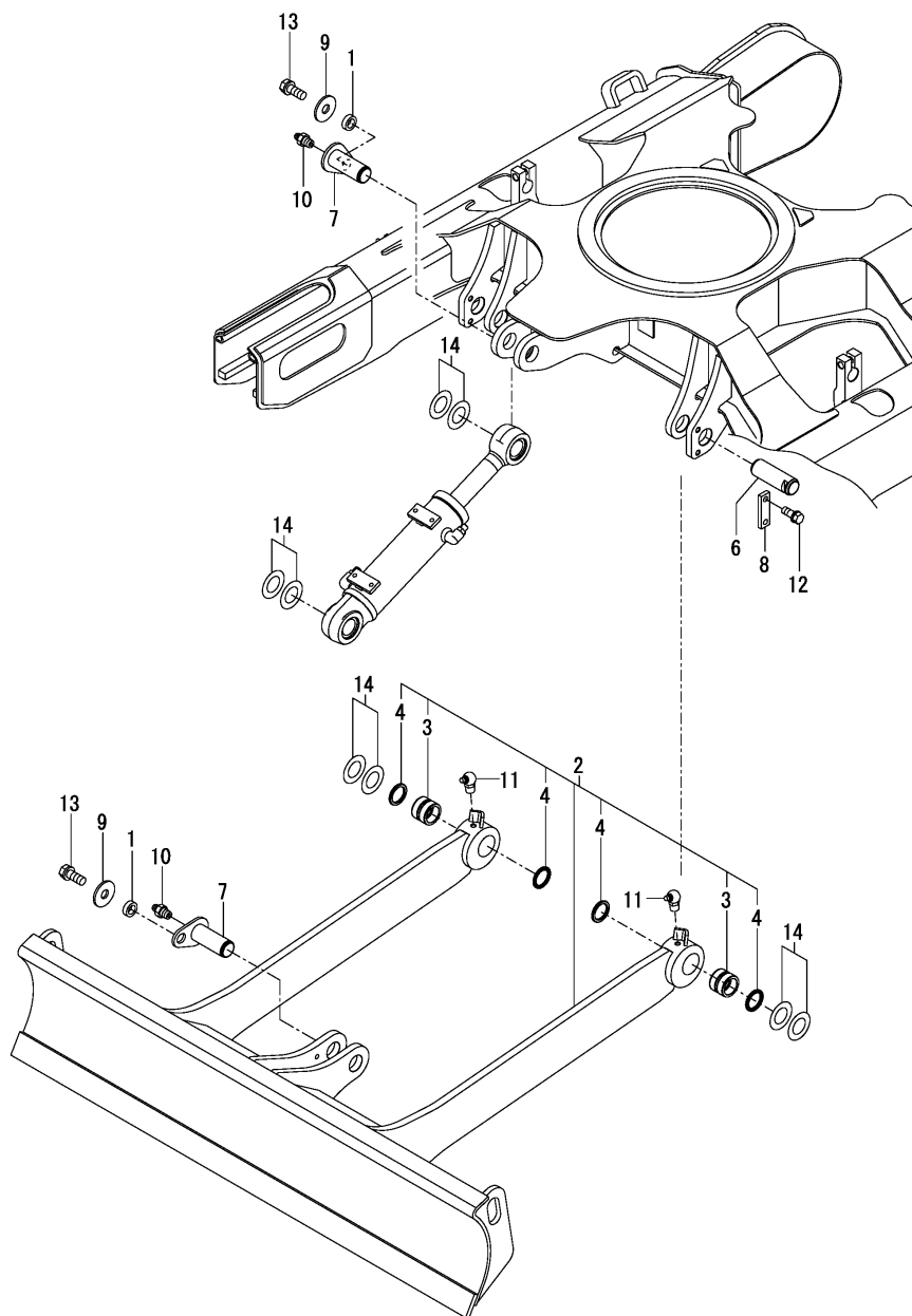
Fig.126. BLADE
