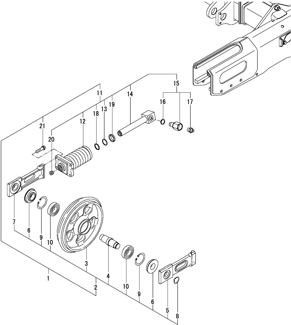
Fig.36. IDLER & ADJUST
