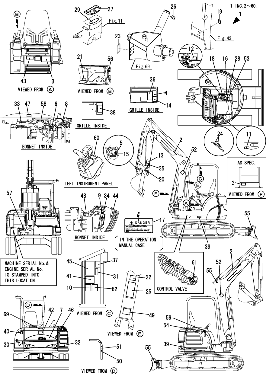
Fig.97. (2A)LABEL(CANOPY)(ANGLE BLADE SPEC.)
