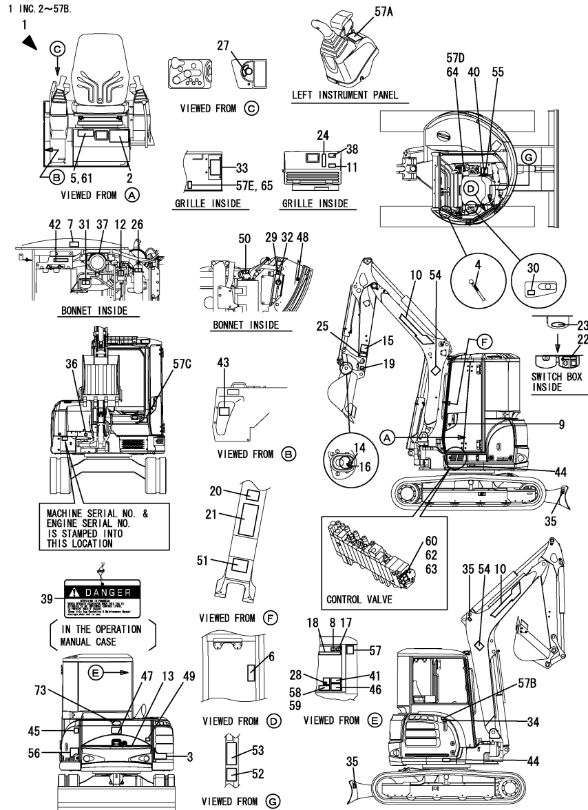
Fig.1. LABEL(CABIN)
